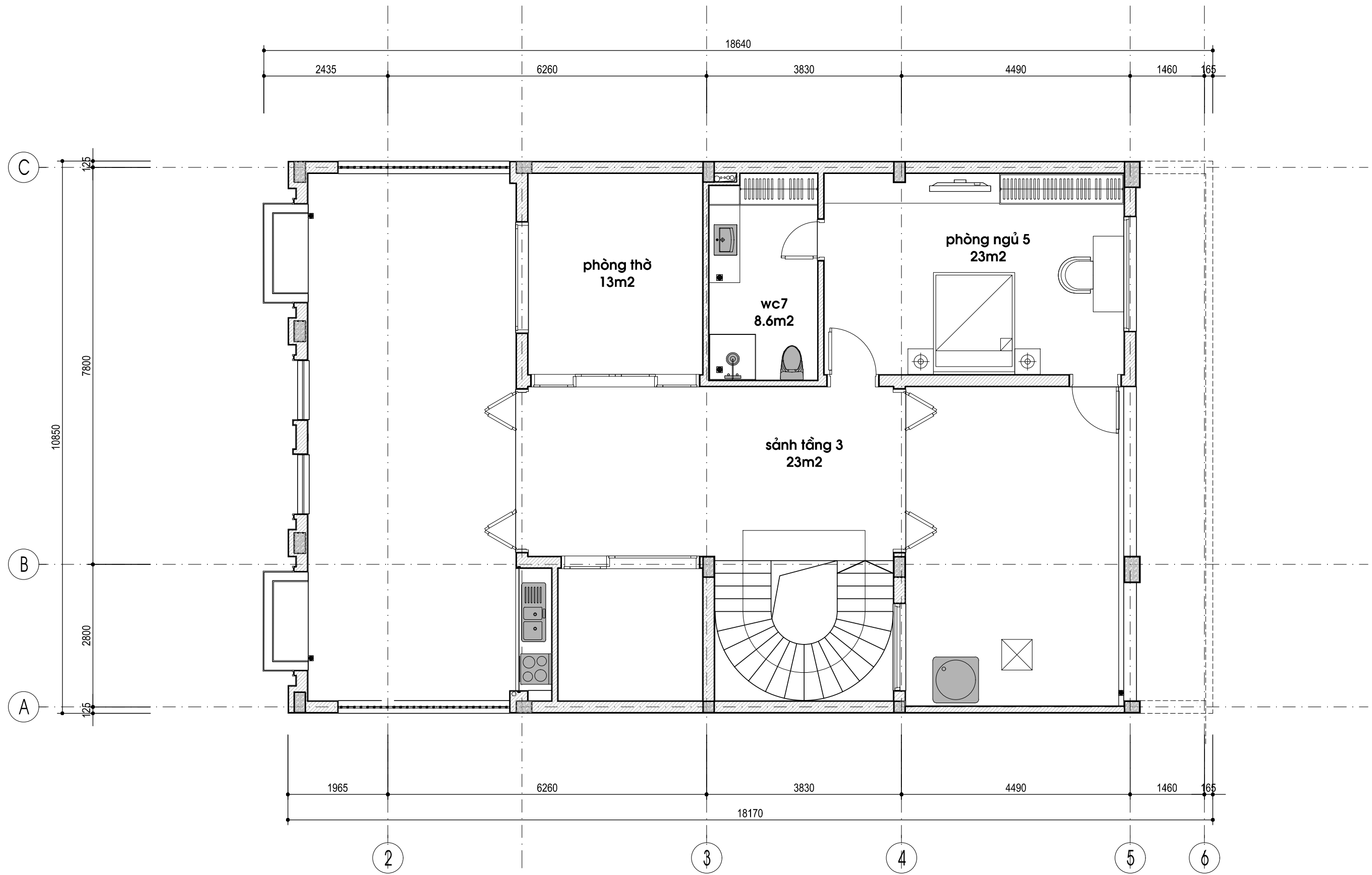
MẶT BẰNG T3
