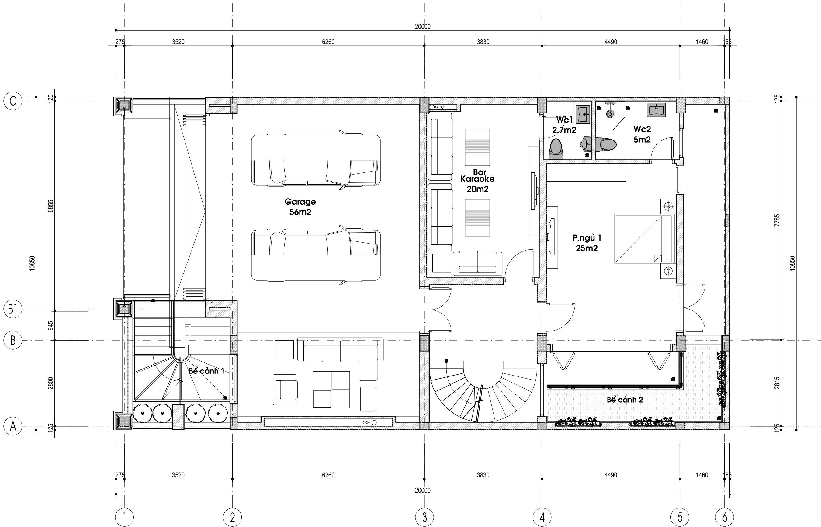
MẶT BẰNG TẦNG TRỆT
