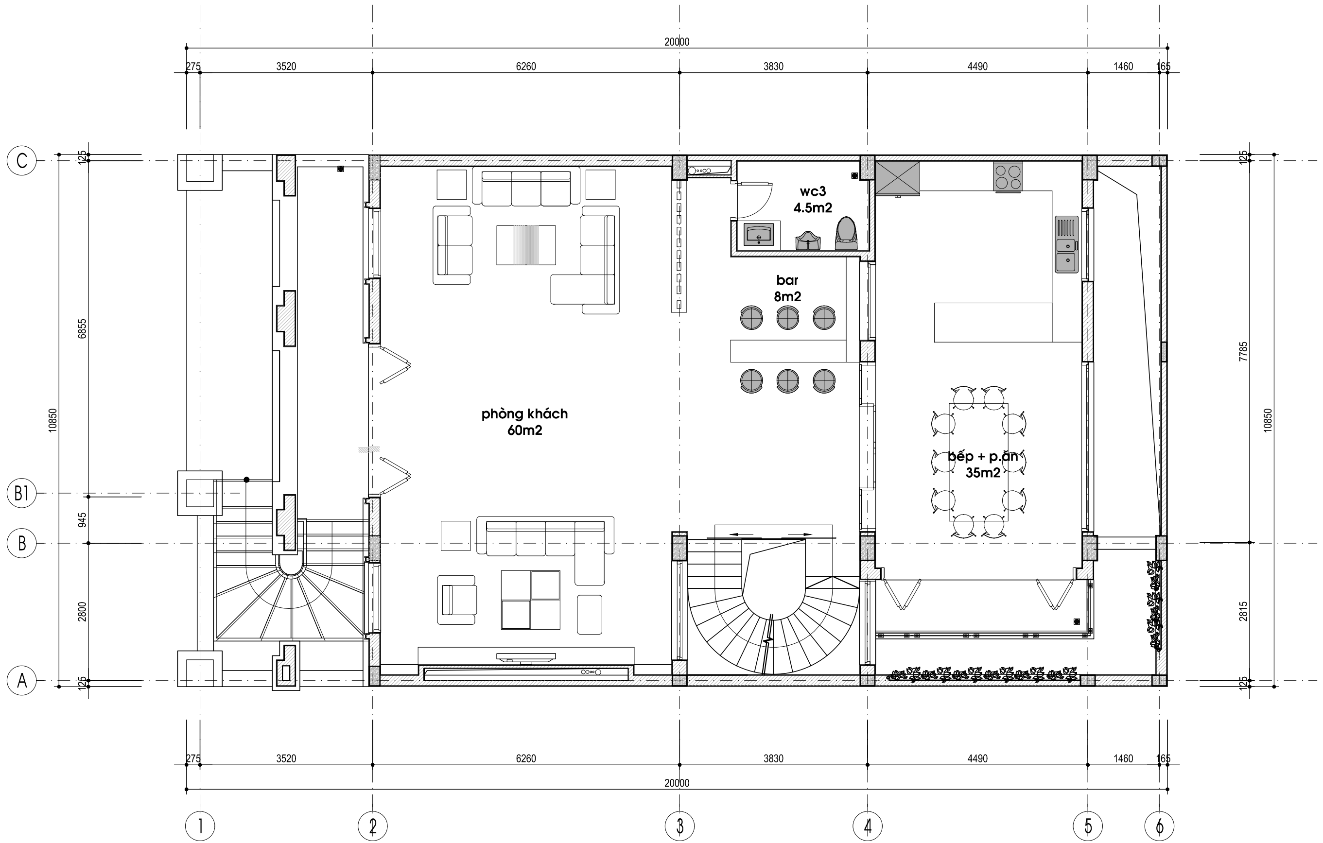
MẶT BẰNG TẦNG 1
